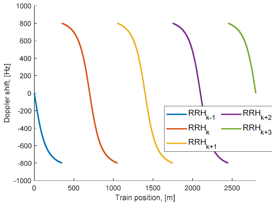
Figure B.3.3-3 Doppler shift trajectory ( f_d
