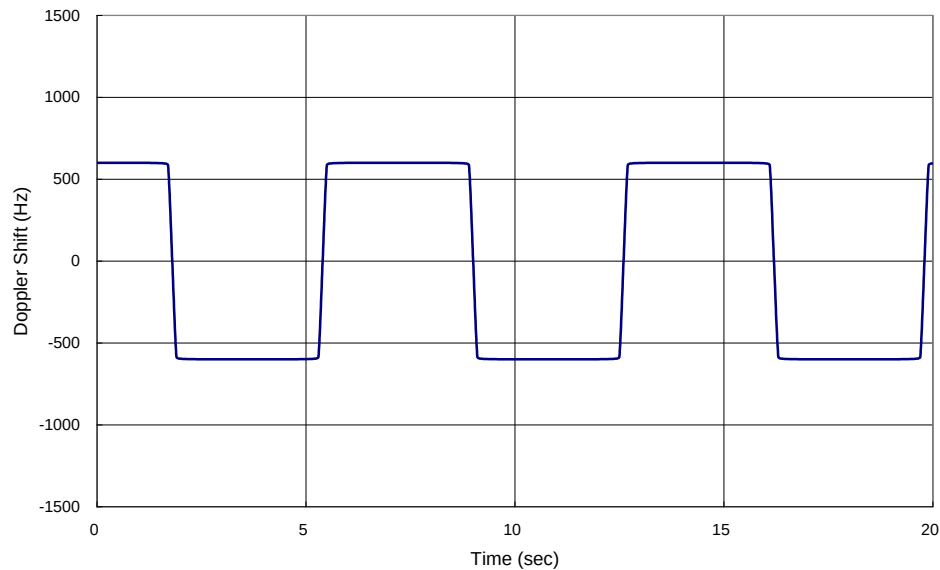
Figure D.2.4A.1: Doppler shift trajectory
