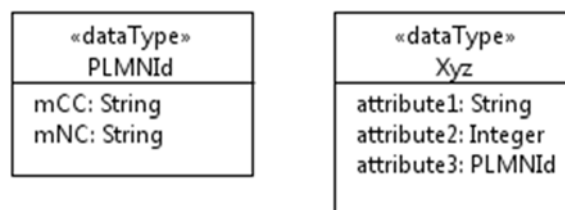
Figure 5.3.4.2-1: <<dataType>> notations
