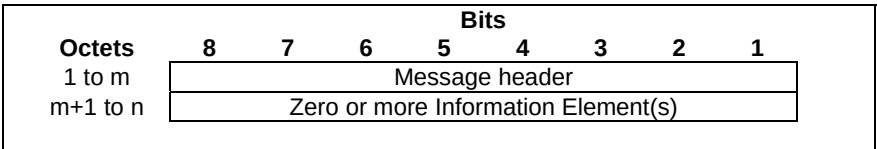
Figure 7.1.2.1-1: Message Format
