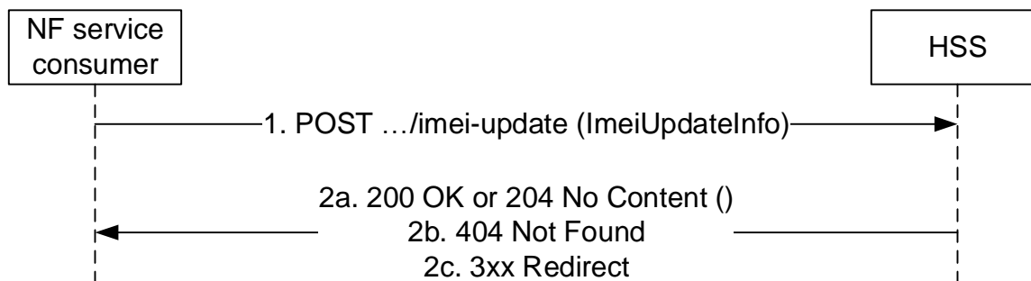
Figure 5.4.2.3-1: IMEI Update
