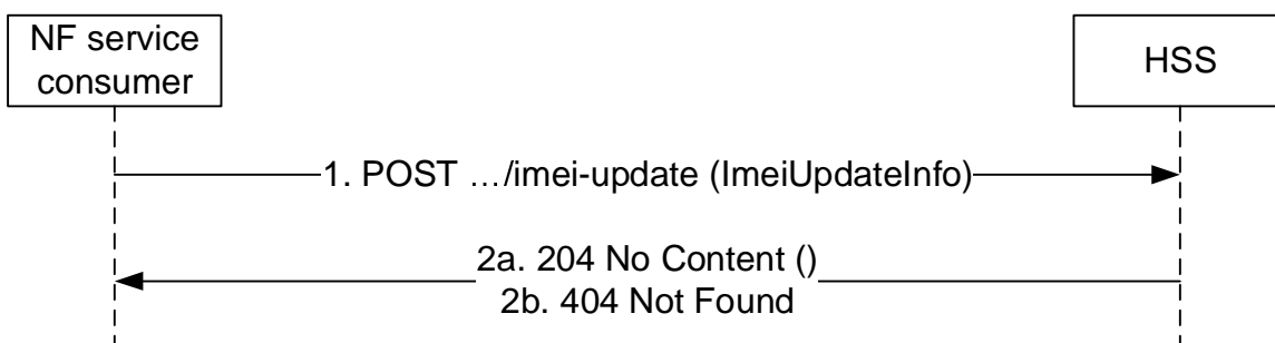
Figure 5.4.2.2.3-1: IMEI Update
