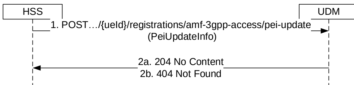
Figure 5.3.2.10.2-1: PEI Update
