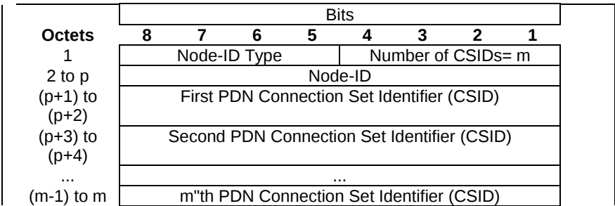
Figure 12.1.1.2-1: FQ-CSID
