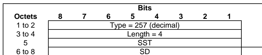
Figure 8.2.176-1: S-NSSAI
