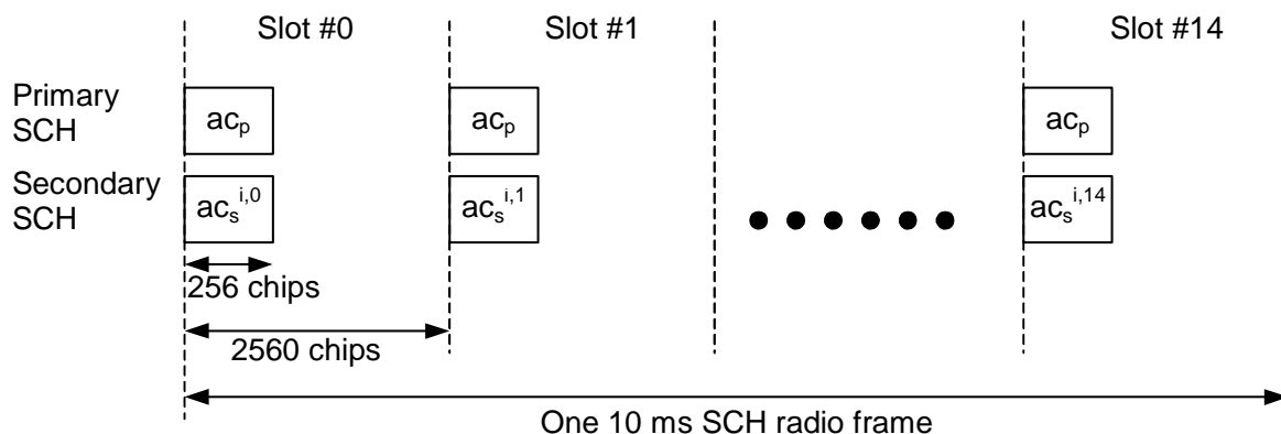
Figure 19: Structure of Synchronisation Channel (SCH)
