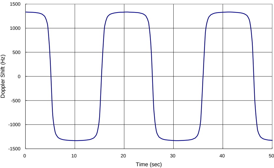
Figure B.3: Doppler shift trajectory for scenario 1
