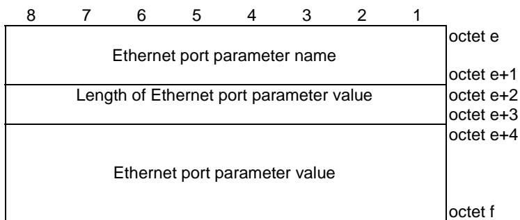
Figure 9.4.3: Ethernet port parameter status
