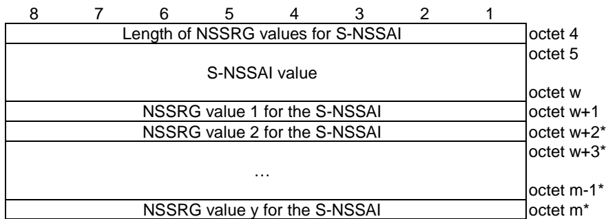
Figure 9.11.3.82.2: NSSRG values for S-NSSAI
