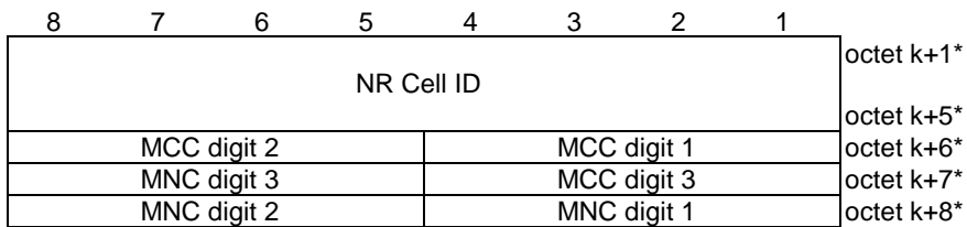
Figure 9.11.4.31.7: NR CGI
