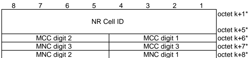
Figure 9.11.4.31.7: NR CGI
