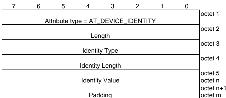
Figure 8.2.8.1-1: AT_DEVICE_IDENTITY attribute
