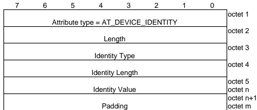
Figure 8.2.8.1-1: AT_DEVICE_IDENTITY attribute
