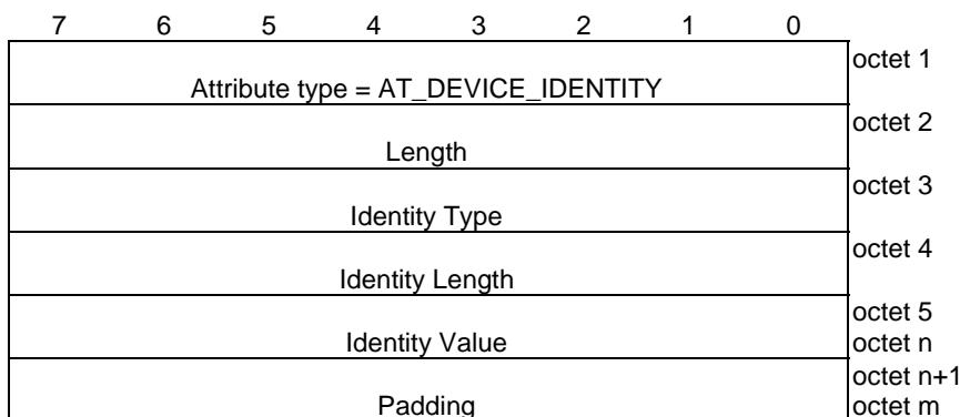
Figure 8.2.8.1-1: AT_DEVICE_IDENTITY attribute
