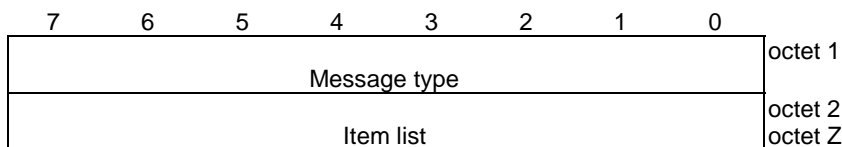
Figure 8.1.4.1-1: Message
