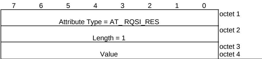
Figure 8.1.1.2-1: AT_RQSI_RES attribute.
