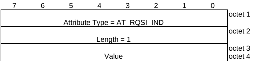
Figure 8.1.1.1-1: AT_RQSI_IND attribute
