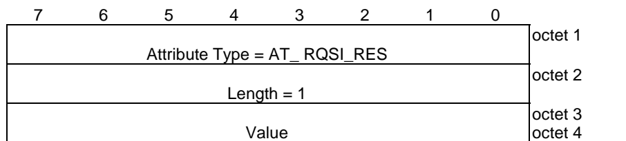
Figure 8.1.1.2-1: AT_RQSI_RES attribute.
