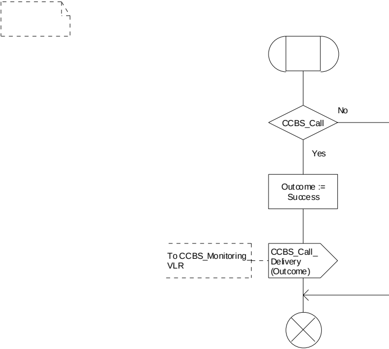
Procedure CCBS_ICH_VLR_Report_Success
