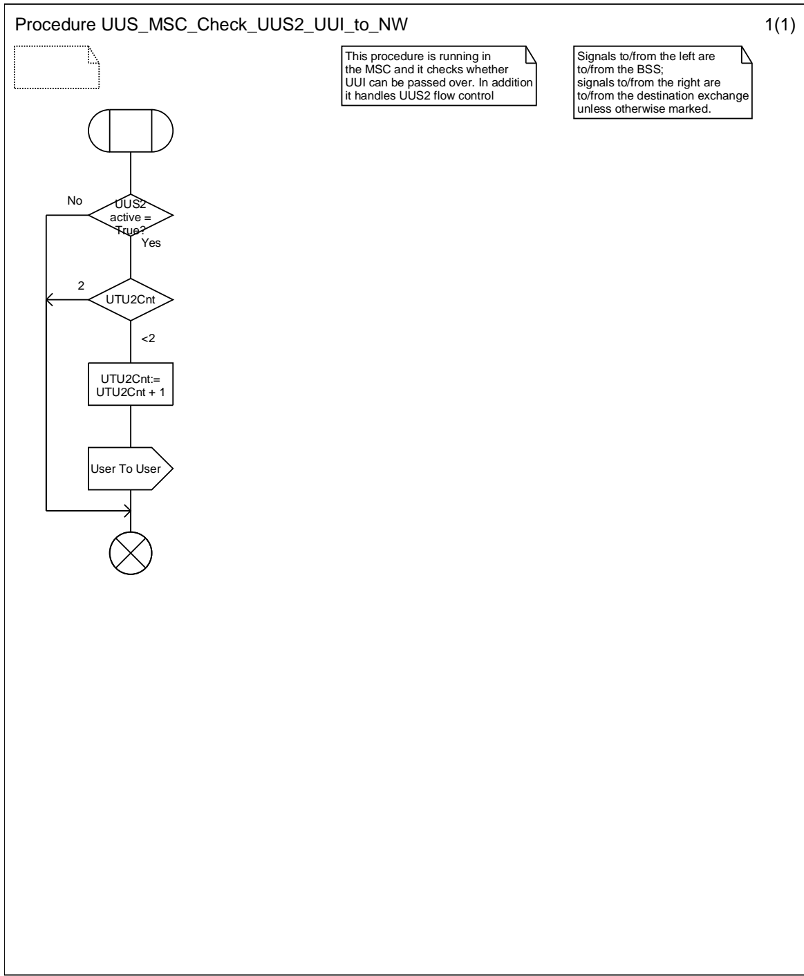
Figure 9.3.3: Procedure UUS_MSC_Check_UUS2_UUI_to_NW
