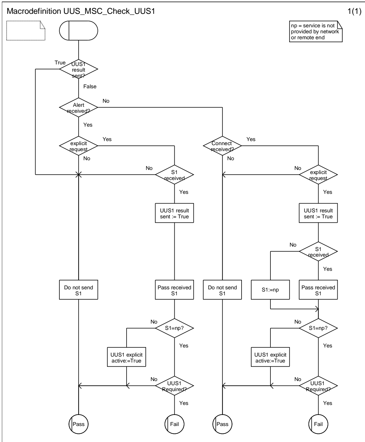
Figure 9.3.7: Macrodefinition UUS_MSC_Check_UUS1
