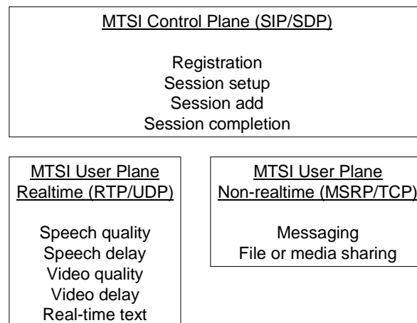
Figure 40: MTSI parameter structure
