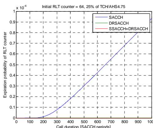
(d) 25% FER of TCH/AHS4.75
