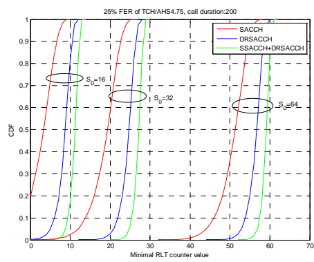
(d) 25% FER of TCH/AHS4.75
