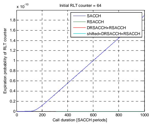
(a) 1% FER of TCH/AFS4.75
