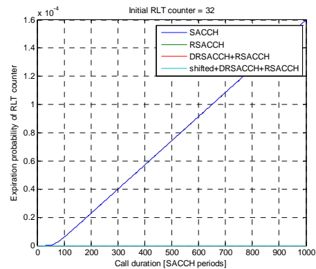
(a) 1% FER of TCH/AFS4.75
