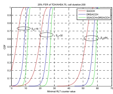
(d) 25% FER of TCH/AHS4.75
