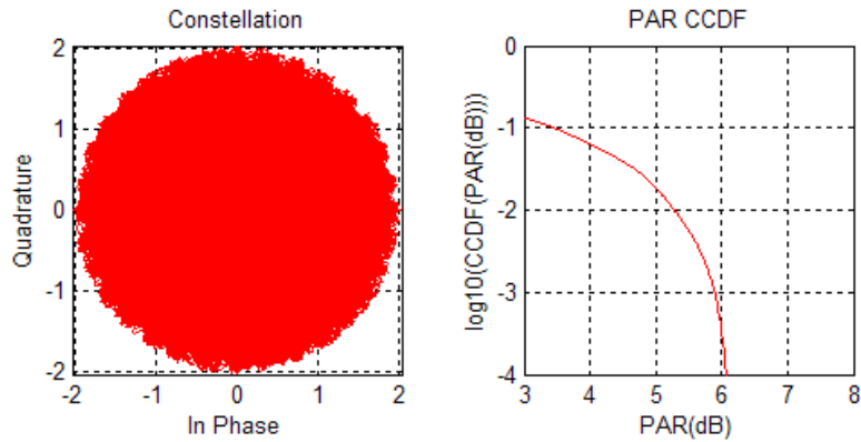
Figure 63: Dual-carrier 8PSK constellation and PAR CDF
