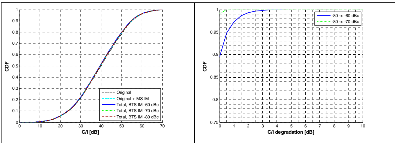
Figure 13. C/I CDF comparing MPCA IM
