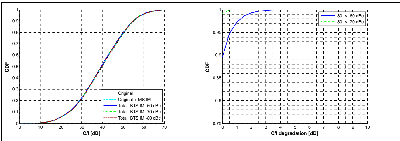
Figure 13. C/I CDF comparing MPCA IM
