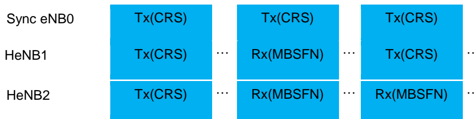
Fig. 6.4.2.1.2-1 Tracking using MBSFN Subframes
