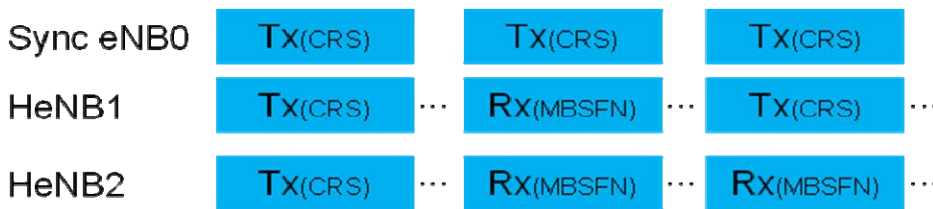
Fig. 6.4.2.1.2-1 Tracking using MBSFN Subframes
