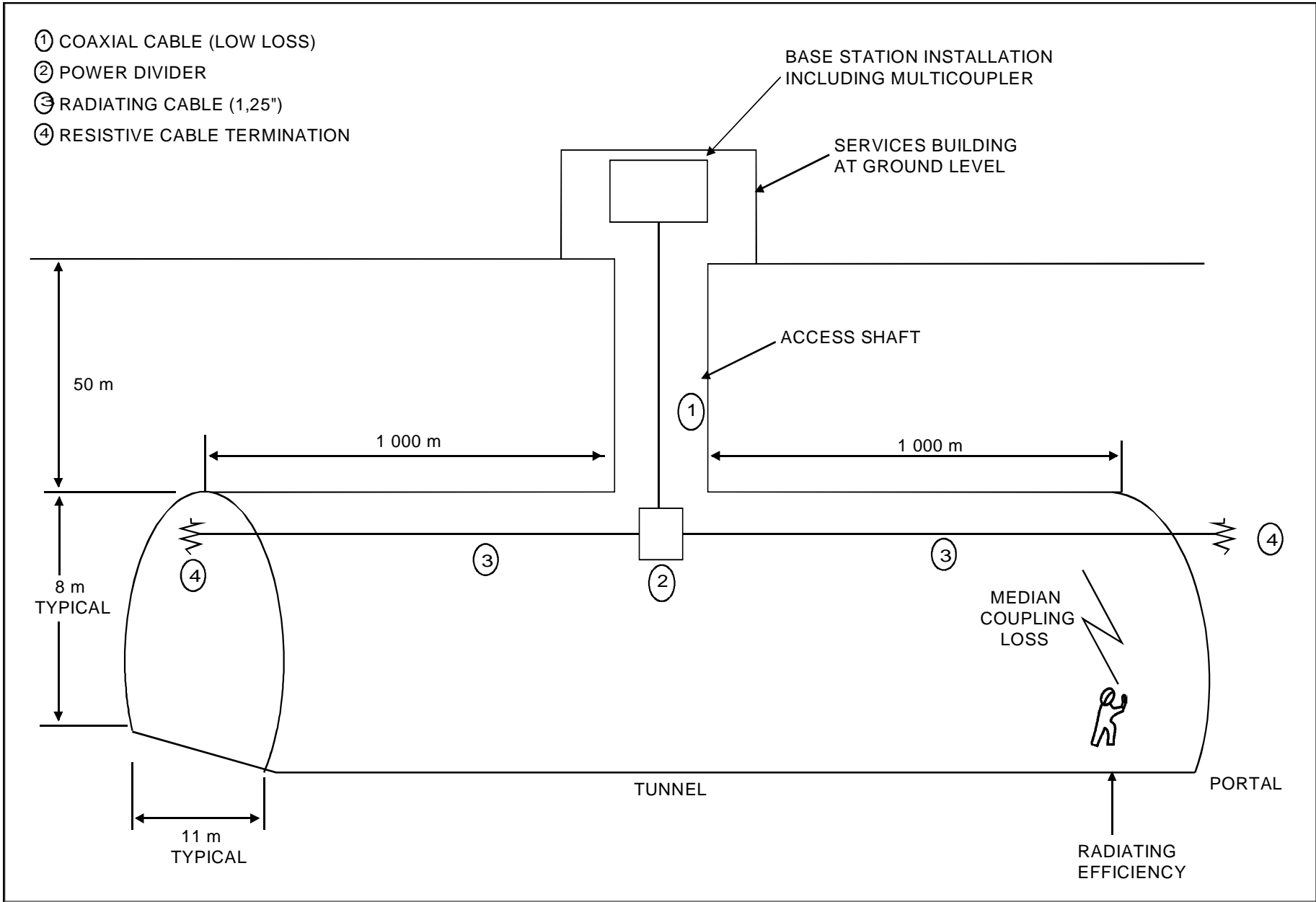
Figure N.1: Typical confined space R.F. system
