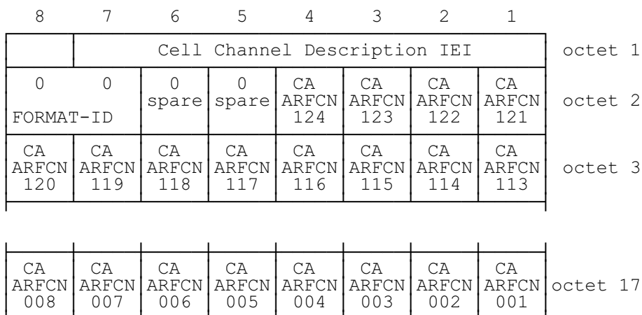
Figure 10.10/GSM 04.08
