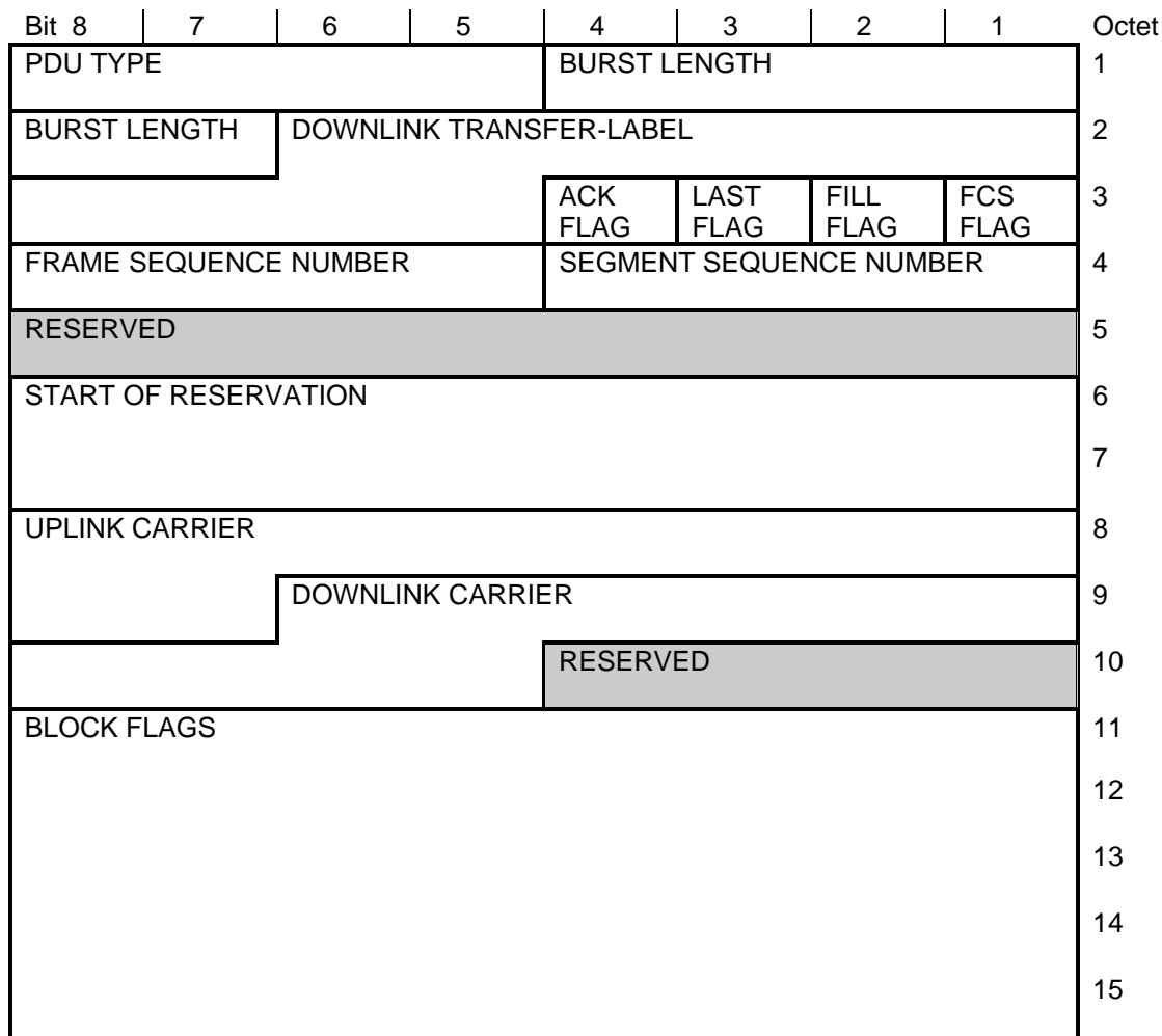
Figure 86: <DD2> PDU
