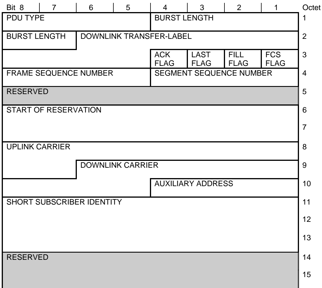
Figure 85: <DD1> PDU
