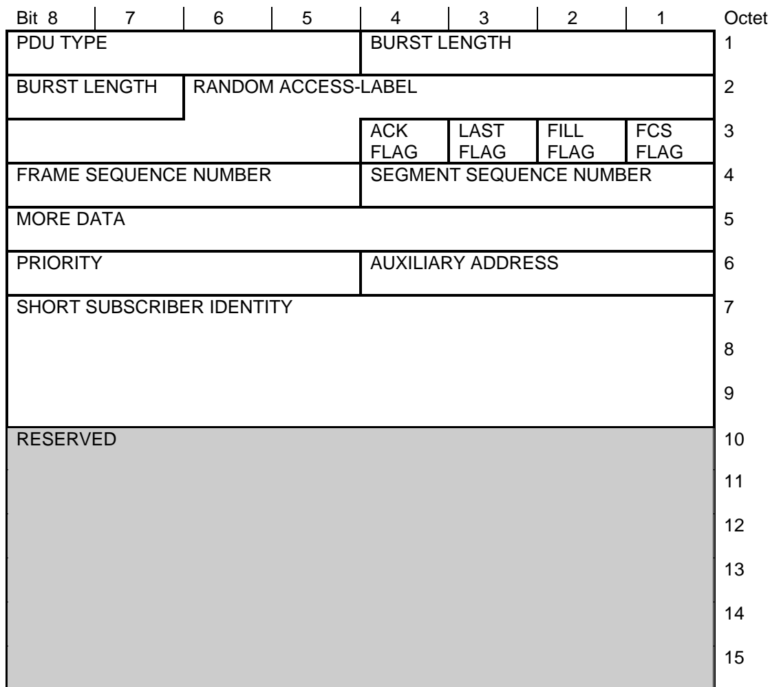
Figure 79: <UD1> PDU
