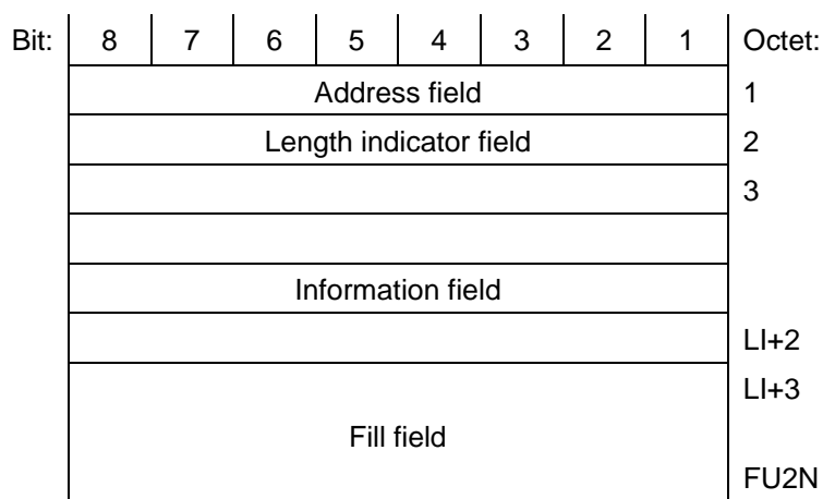
Frame Format Type FU2
