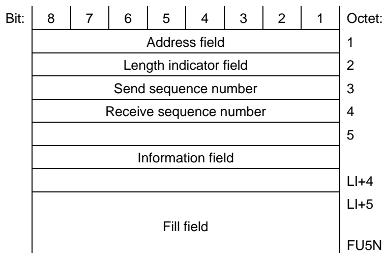
Frame format type FU5a
