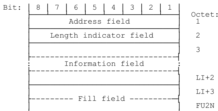
Frame Format Type FU2
