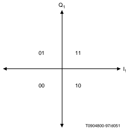
Figure N.1: QPSK symbol mapping
