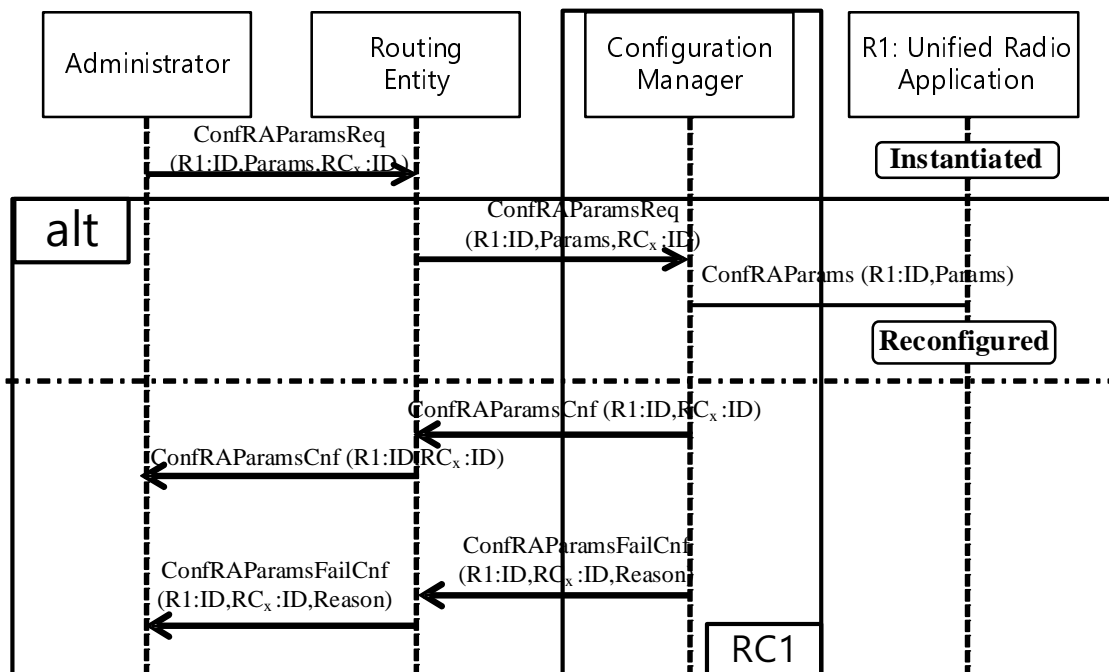
Figure 6.2.2-1: Configuring URA parameters
