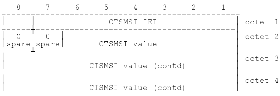
Figure 10.1/GSM 04.56 CTSMIS information element
