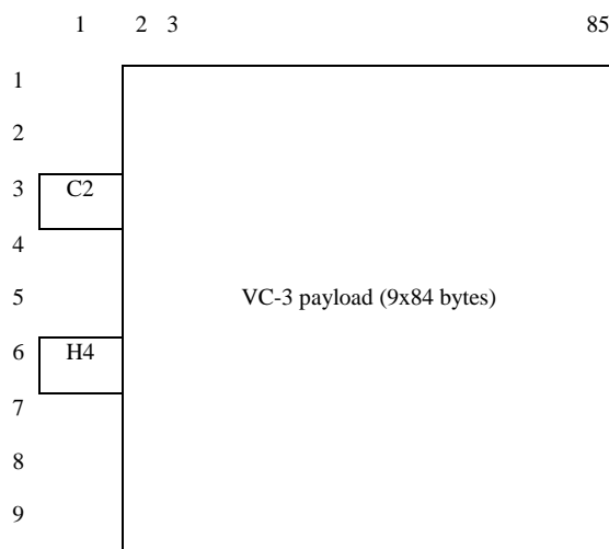
Figure 89: S3/TSS3_AI_So_D
