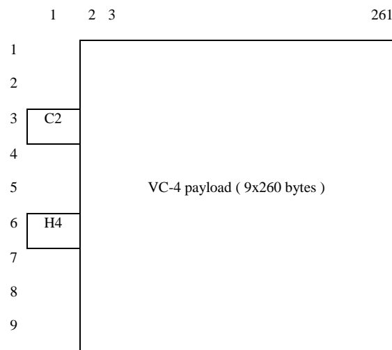
Figure 49: S4/TSS1_AI_So_D
