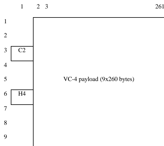
Figure 13: S4/P4x_AI_So_D
