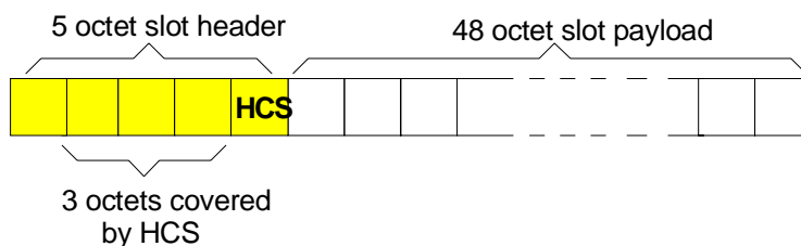
Figure 45: DQDB slot format
