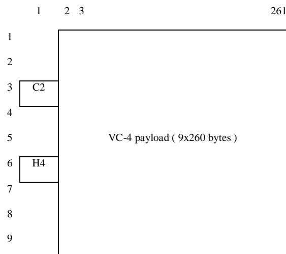
Figure 49: S4/TSS1_AI_So_D
