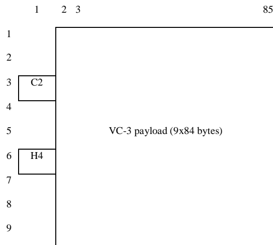
Figure 89: S3/TSS3_AI_So_D
