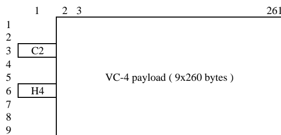
Figure 13: S4/P4x_AI_So_D
