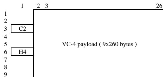
Figure 49: S4/TSS1_AI_So_D
