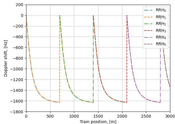
Figure B.3.6-4 Doppler shift trajectories ( f_d = 1667 Hz)
