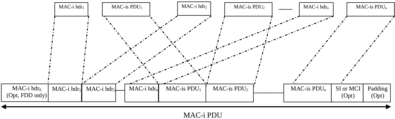
Figure 9.1.5-4a: MAC-i PDU.
