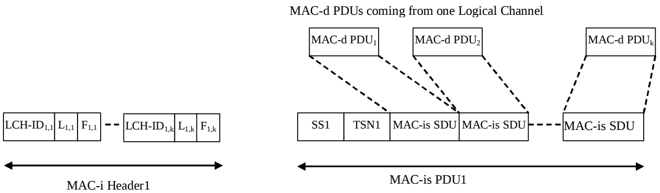
Figure 9.1.5-3 MAC-is PDU.
