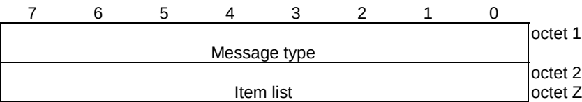
Figure 8.1.4.1-1: Message
