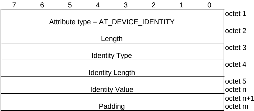
Figure 8.2.8.1-1: AT_DEVICE_IDENTITY attribute
