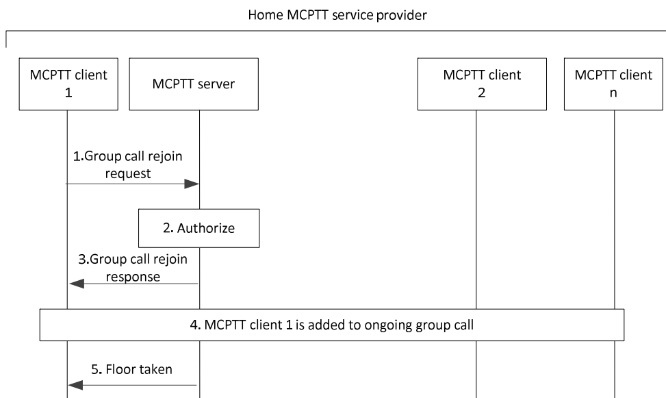
Figure 10.6.2.3.1.1.5-1: Rejoin call
