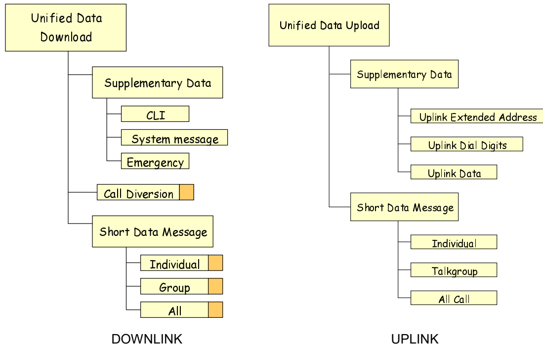
Figure 5.7: UDT Header
