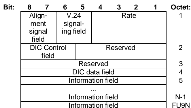
Figure 11.11.1.1.1.1: Frame Format Type FU9
