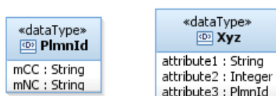
Figure 5.3.4.2-1: &lt;&lt;dataType&gt;&gt; notations
